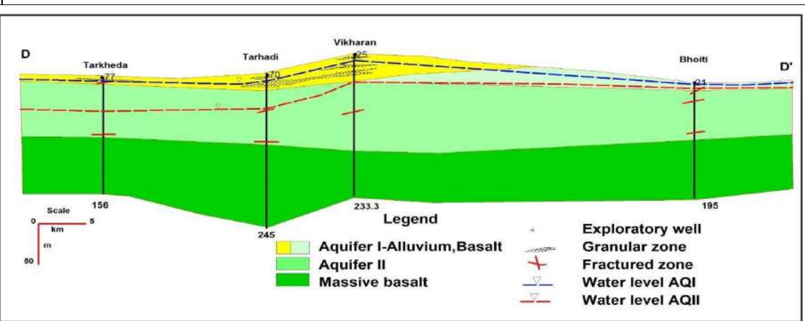
Figure 2.9 (d): Lithological section
